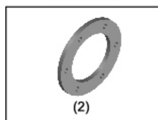
PD8020 SLIPPER FRICTION RINGS 限滑來令片
