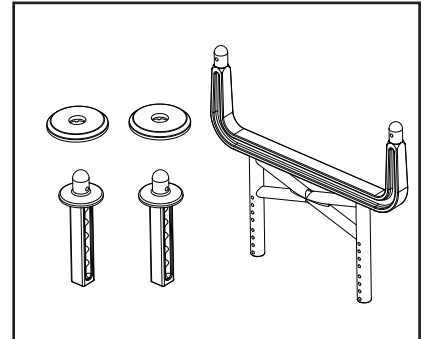
PD90453S1 Rear Body Post 後車殼支柱
