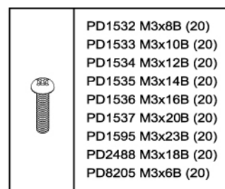
BHPS SCREW 圓頭十字螺絲
