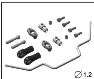
PD9200-1 SWAY BAR SET(SILVER) 防傾桿組(銀)
