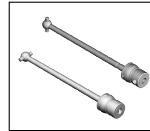
PD1872 CTR CVA FR/RR,S3
