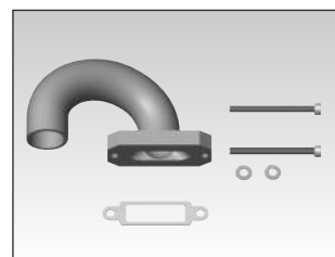
PN1527 MANIFOLD, 50 PIPE 排氣彎管組
