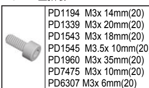
SK H.M SCREW 內六角螺絲
