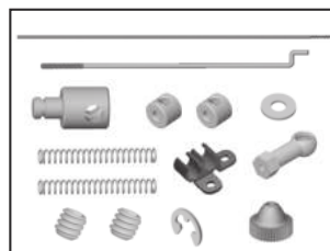
PD7248 THROTTLE/BRAKE LINKAGE 油門&煞車拉桿組
