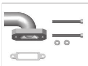
PN1526 MANIFOLD 排氣彎管組
